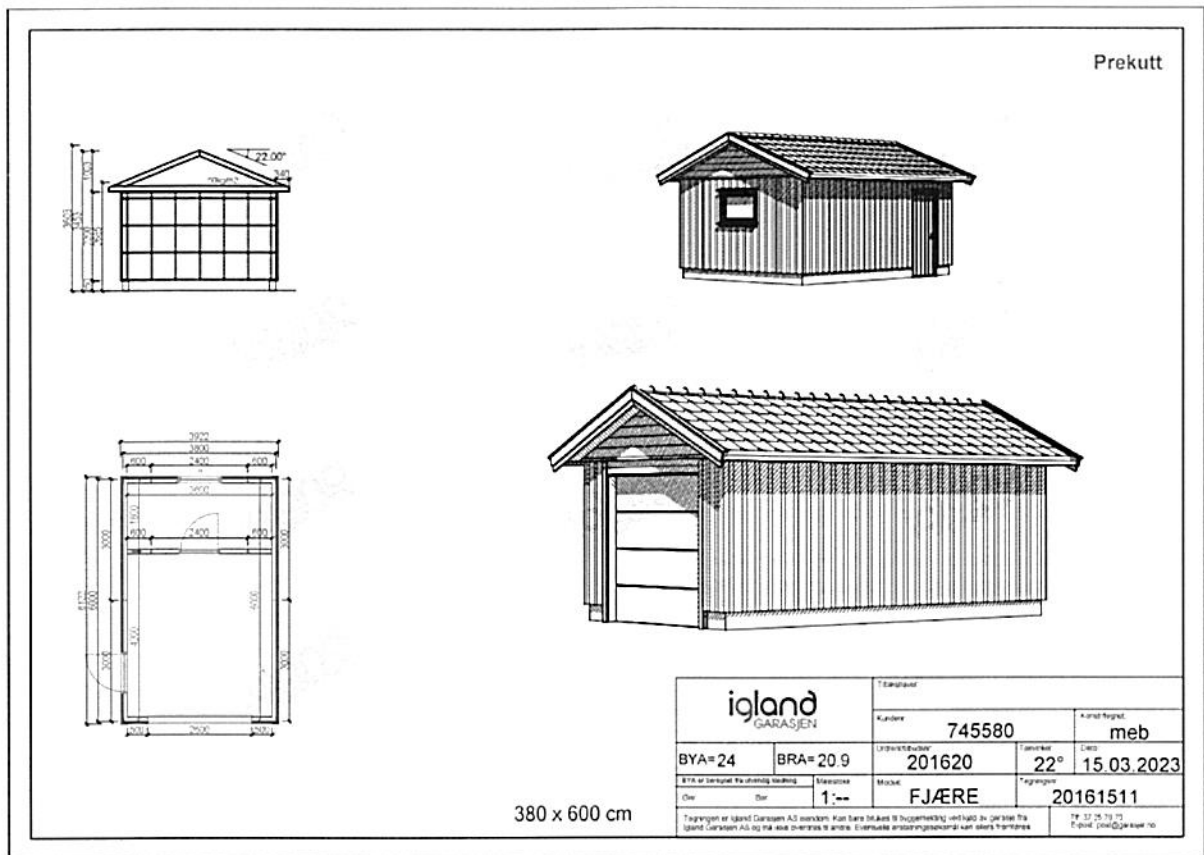
Figur 3. Tegning tilbudt garasje fra Igland.
