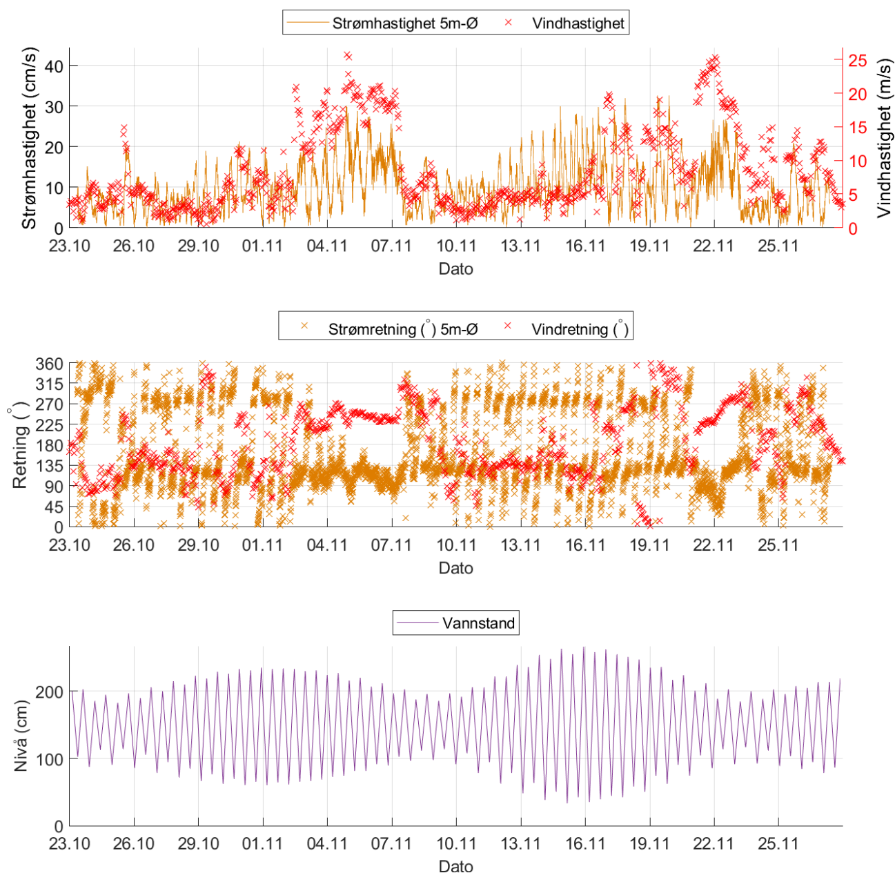
Figur 4.25.3. Strømhastighet (mot retning) på 5m dyp i østlig riggposisjon og vindhastighet (fra retning) på Veiholmen, strøm- og vindretning, samt vannstand (Kristiansund) under måleperioden. Tidspunkter hvor strøm og vind har omtrent motsatt rettet retning indikerer tilfeller med vindpåvirket strøm.
