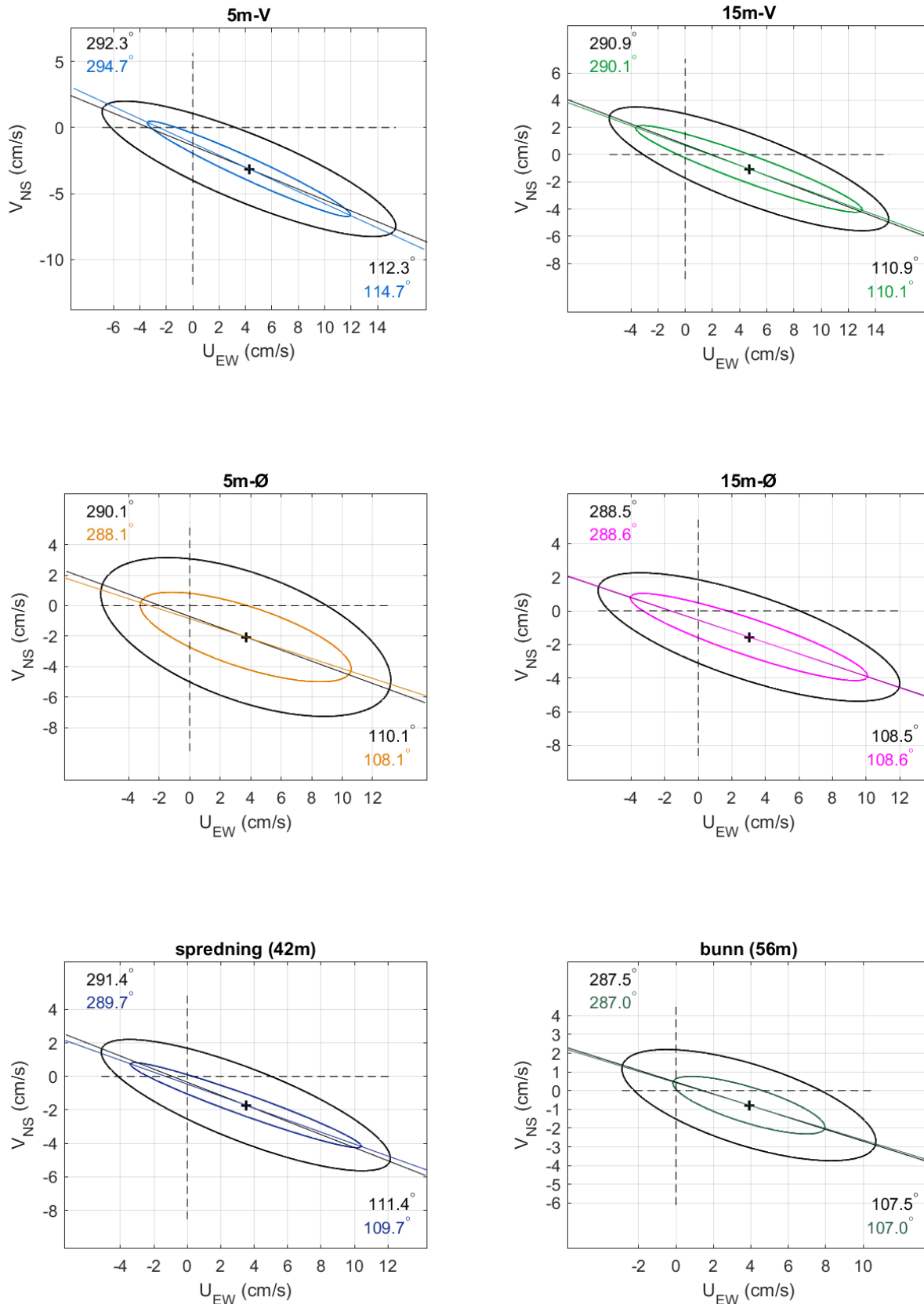
Figur 4.23.2. U_{EW} – V_{NS} tidevannsellipse (farget linje) vist sammen med strørellipsen (svart linje). Midtpunktet for strørellipsene er markert med kryss som også markerer den effektive transporthastigheten. Vinklene indikerer de store halvaksenes orientering i forhold til nord/sør. Aksekor for øst – vest og nord – sør er vist med stiplede linjer.
