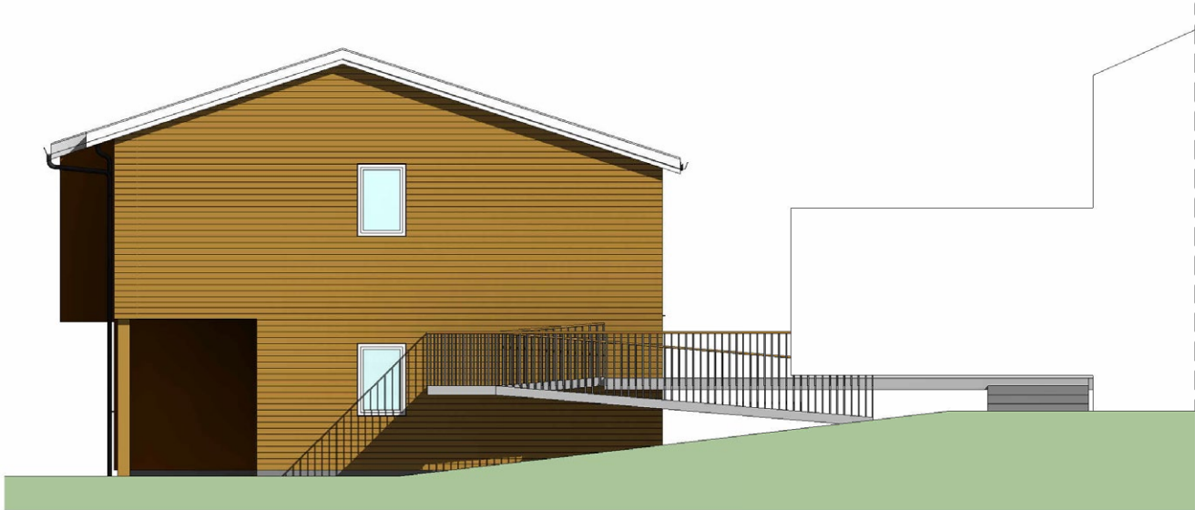
Fasade Øst
