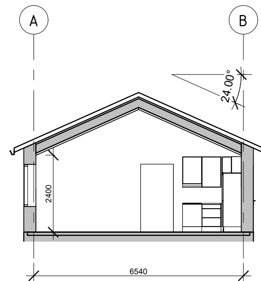
Snitt B
