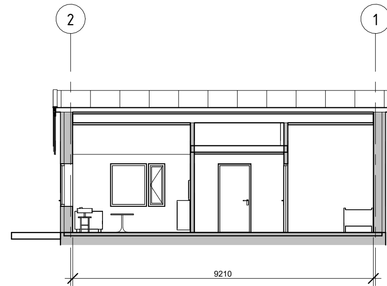
Snitt B
